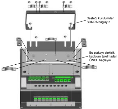
Şekil 6: PE'nin (plaka ve API kablo desteği) bağlanması, MI4 - MI5
