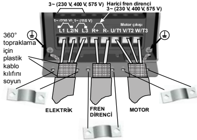
Şekil 8: Vacon 20 elektrik bağlantıları, MI2 - MI3
