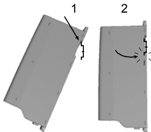
Şekil 3: DIN-rama montaj, MI1 - MI3
