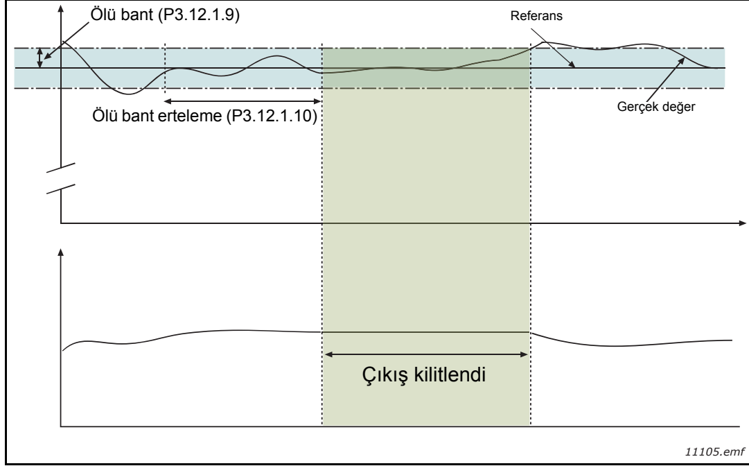
Şekil 33. Ölü bant
