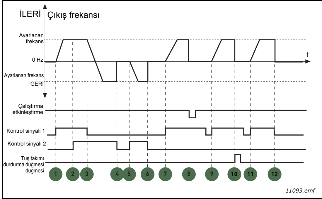
Şekil 21. G/Ç A Başlat/durdur mantığı = 2
