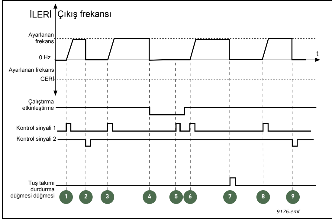
Şekil 20. G/Ç A Başlat/durdur mantığı = 1
