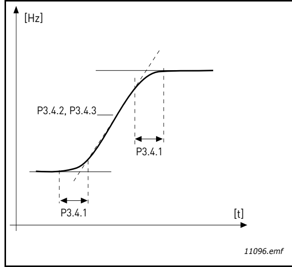
Şekil 24. Hızlanma/Yavaşlama (S-şekilli)
