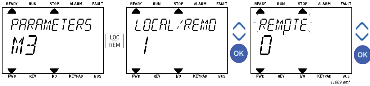
Şekil 10. Kontrol yeri değiştirilmesi
